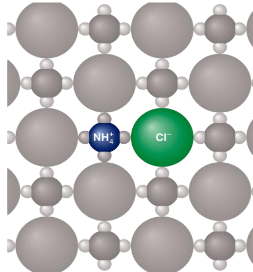
Cloruro di ammonio \text{NH}_4\text{Cl}
