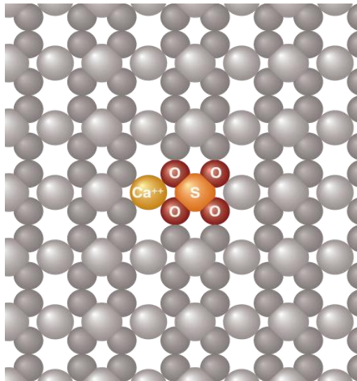
Solfato di calcio \text{CaSO}_4
